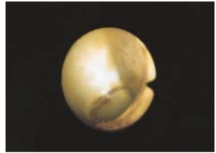
106号室PS内 部位:戸別配管 内視鏡ファイバースコープによる映像 わずかに異種金属接合部にこぶ錆が発生
