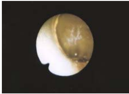
106号室PS内 部位:戸別配管 内視鏡ファイバースコープによる映像 わずかに異種金属接合部にこぶ錆が発生
